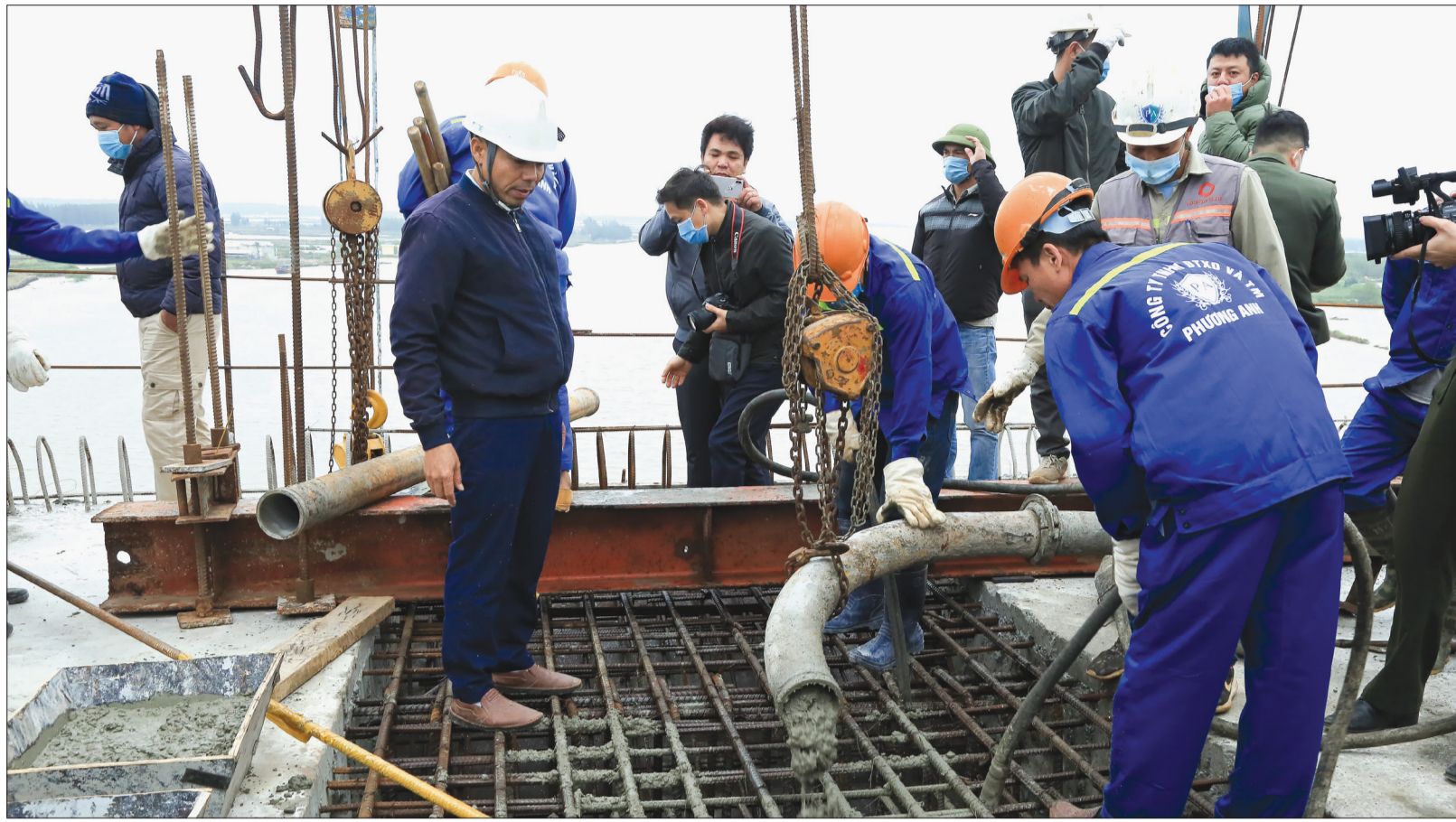
Công nhân Công ty TNHH Đầu tư xây dựng và thương mại Phương Anh đổ bê tông hợp long cầu vượt sông Trà Lý.
