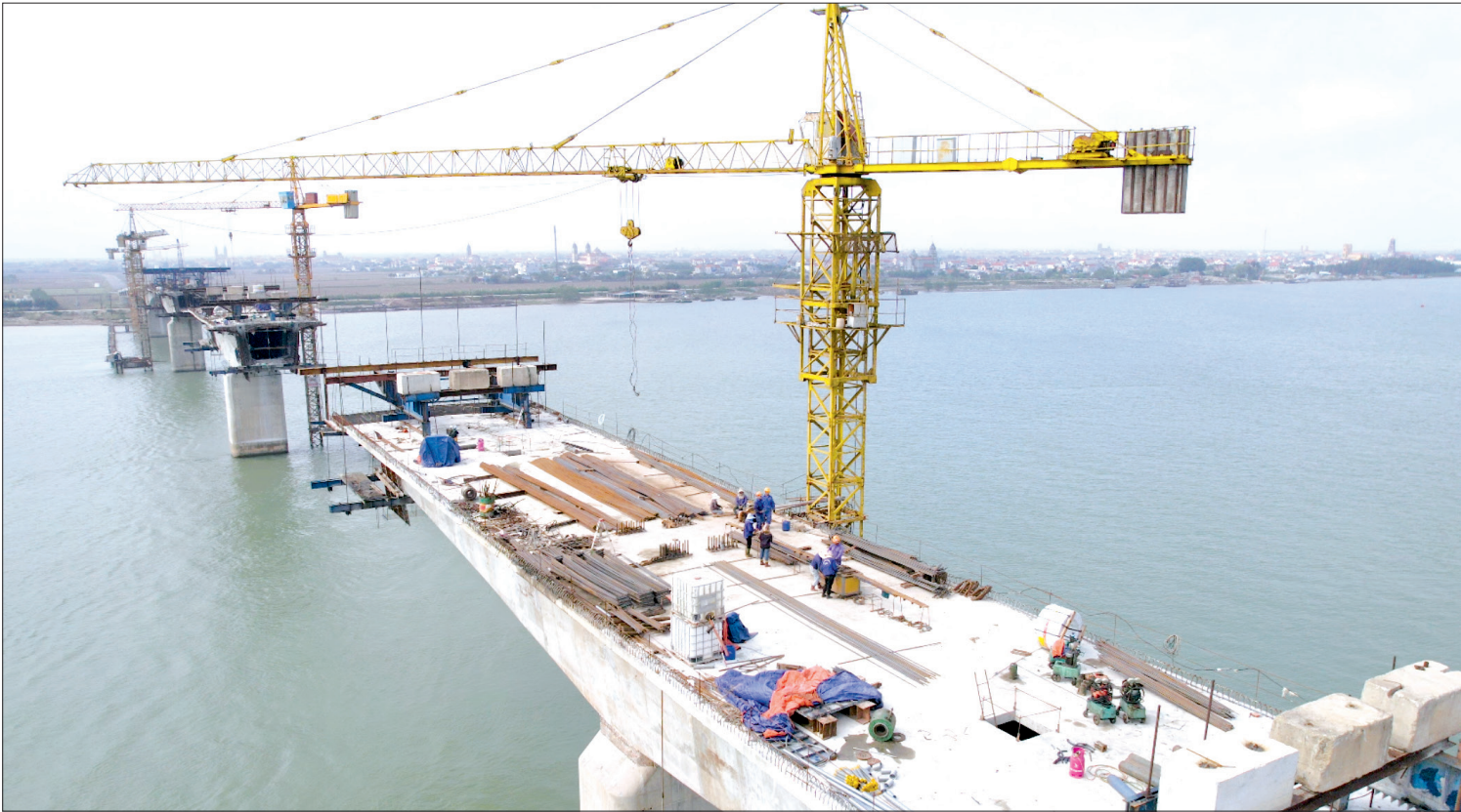
Công trình cầu sông Hồng thuộc tuyến đường bộ ven biển đang dần hoàn thiện.
