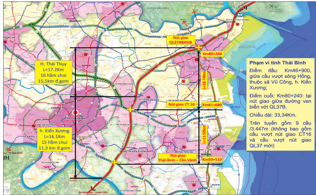
Hướng tuyến của cao tốc CT.08, đoạn qua tỉnh Thái Bình.
