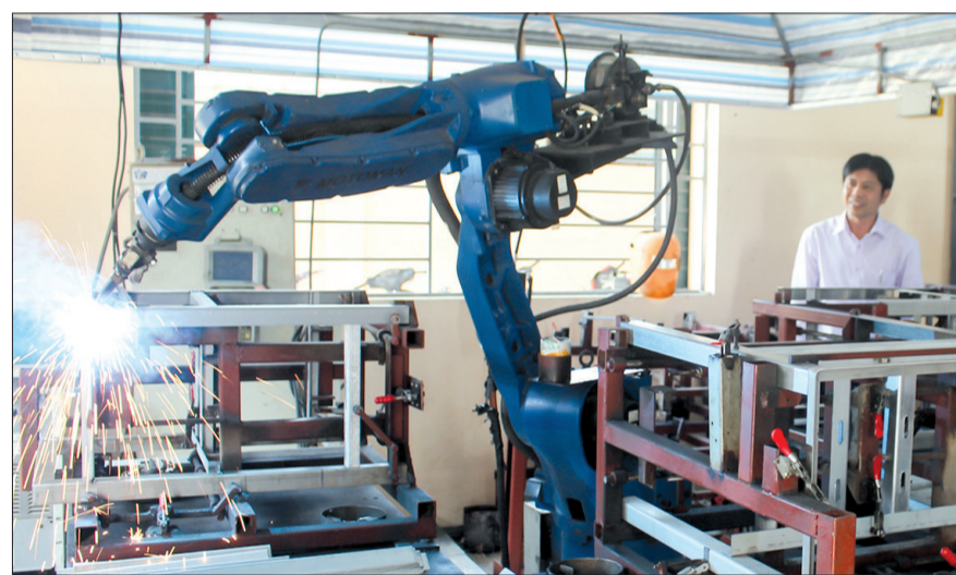
Cánh tay rô bốt thực hiện công đoạn hàn tại Doanh nghiệp tư nhân điện cơ Thiên Thuận.
