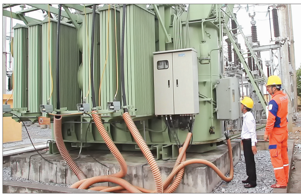
Công nhân Điện lực Kiến Xương kiểm tra trạm biến áp.
